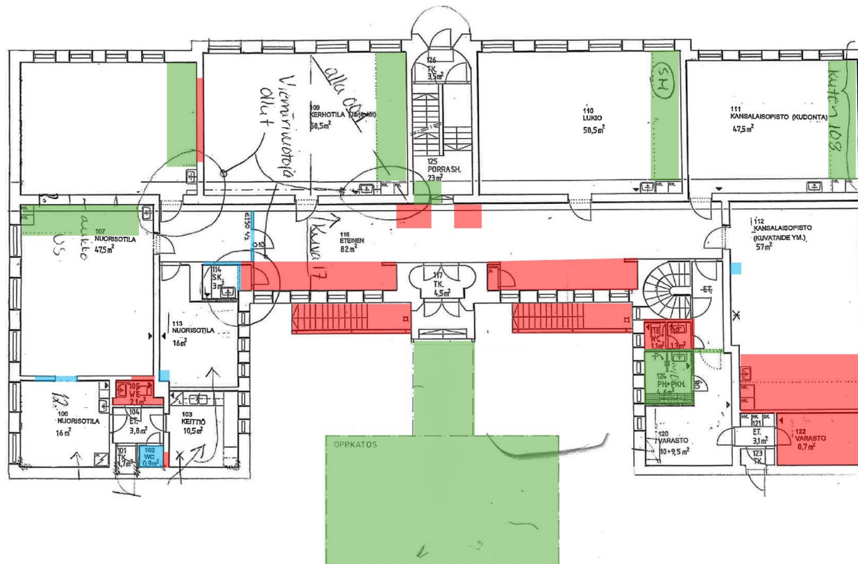
Kuva 43 Vanhan kansakoulurakennuksen maantasokerros. 1960-luvulla tehdyt muutokset korostettu kuvaan punaisella värillä, 1980-luvulla tehdyt muutokset korostettu kuvaan vihreällä värillä, ja 2000-luvulla tehdyt muutokset korostettu kuvaan sinisellä värillä. Taustalla tuorein pohjapiirros vuodelta 2005.
